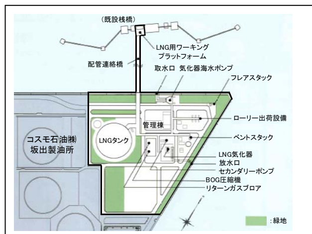
図-2 坂出 LNG 基地全体平面図
